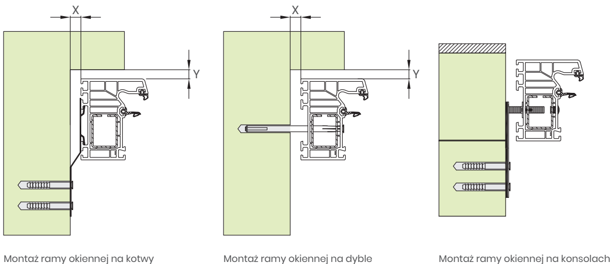
Rys. 5. Rodzaje łączników mechanicznych.
