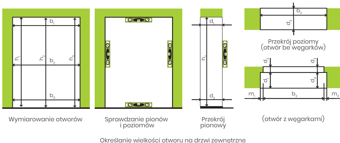
Rys. 3. Wymiarowanie ościeża w ścianie: bez węgarka, z węgarkiem.
