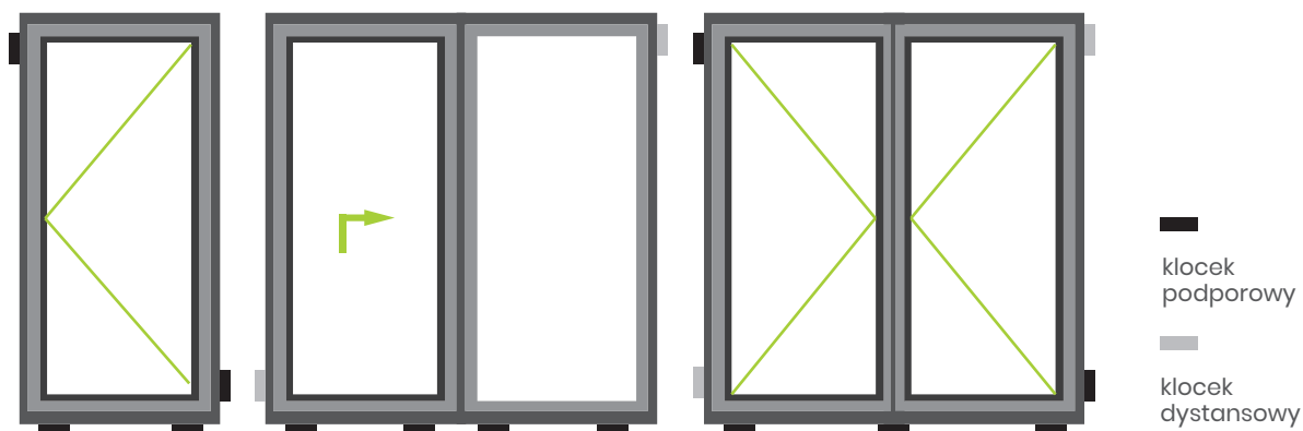
Rys. 2. Usytuowanie klocków / klinów dystansowych do ustalenia pozycji stolarki.
