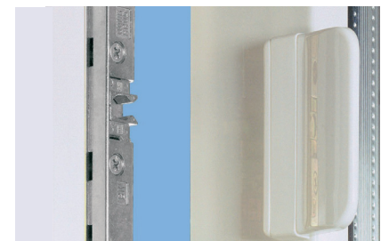
BALKON DEURHENSEL EN SLUITING Hiermee kunt u de deur sluiten door aan de speciale hendel te trekken. De sluiting houdt de vleugel in het kozijn, waardoor tocht, het tegen de kozijn stoten en onbedoeld openen worden voorkomen.
