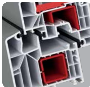
system trzech uszczelnień gwarantuje doskonałą izolację akustyczną i cieplną
